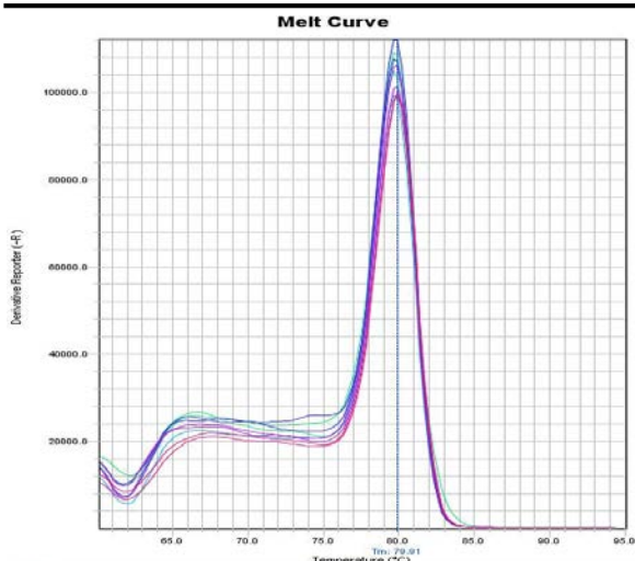
نمودار ۵. منحنی ذوب ژن BCL-XL با نقطه ذوب 79/91°C
