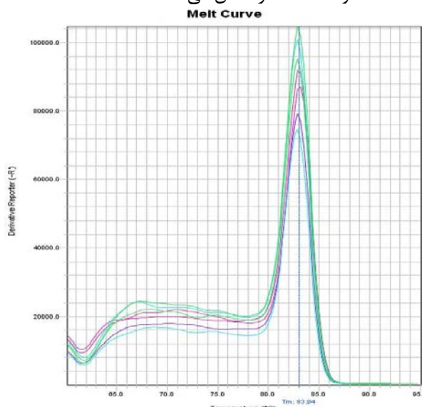
نمودار ۴. منحنی ذوب ژن GAPDH با نقطه ذوب 83/04°C
