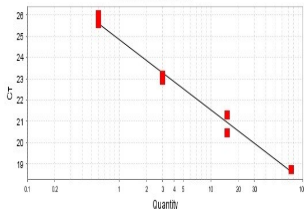
نمودار ۳. منحنی استاندارد ژن GAPDH شیب خط = -۳/۳۳۹ بازده: ۰/۹۹
